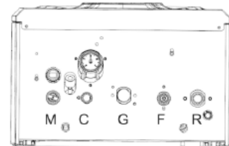
Вид снизу
